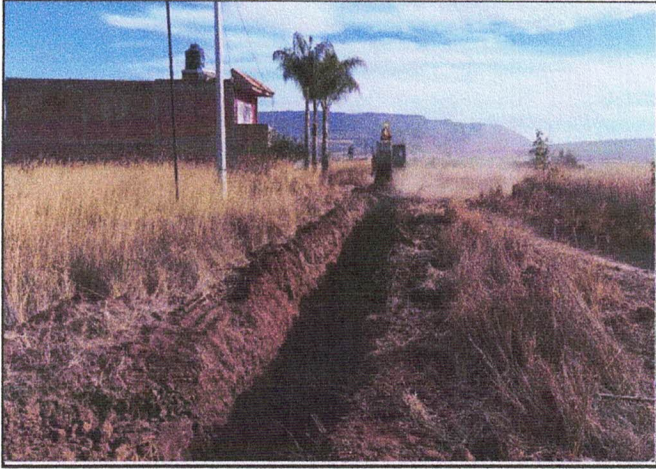
EXCAVACIÓN DE ZANJA PARA COLOCACIÓN DE TUBERÍA.
