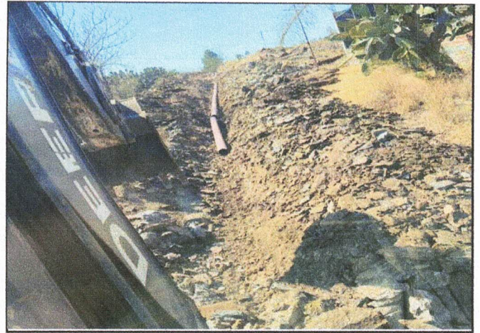
COLOCACIÓN DE TUBERIA SANITARIA PVC DE 10"
